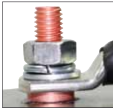
Anwendungsbeispiel Massebolzen / Schaltanlagen
